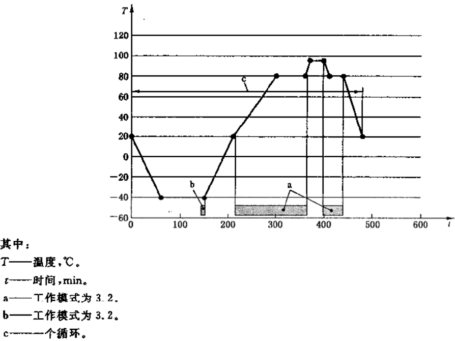
图 3 热浸透阶段温度循环示例(按表 1 代码 F 为例)
